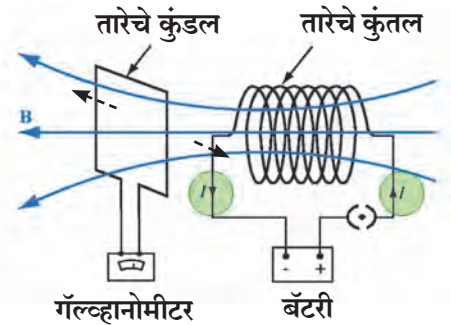
4.16 (ब) कुंडलातून विद्युतधारा प्रवाहित होत असताना कुंडल कुंडलाच्या अक्षाला लंबरेषेत हलविल्यास
