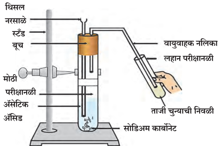
9.24 ऑसेटिक आम्ल व सोडिअम कार्बोनेट यांची अभिक्रिया
