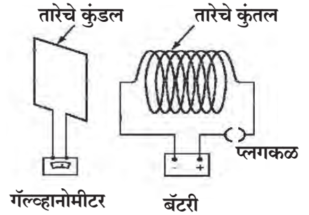
4.16 (अ) कुंडलातून विद्युतधारा प्रवाहित अथवा खंडीत केल्यास
